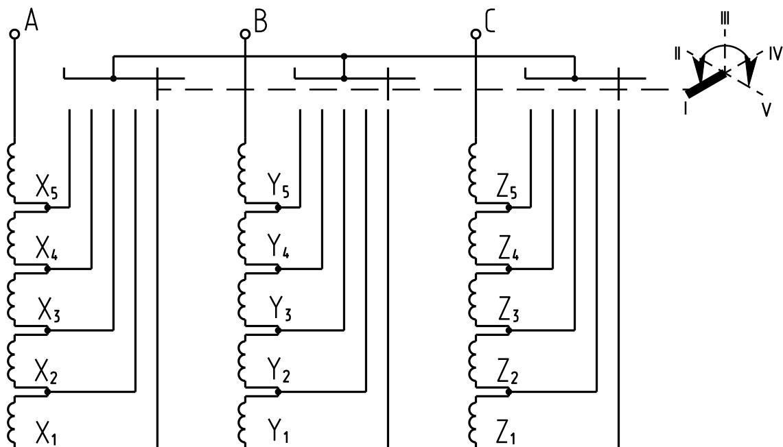
Рисунок 9 – Схема подсоединения ответвлений обмоток ВН к переключателю в трансформаторах мощностью 400 кВ·А при схеме соединения обмоток – «ЗВЕЗДА»
