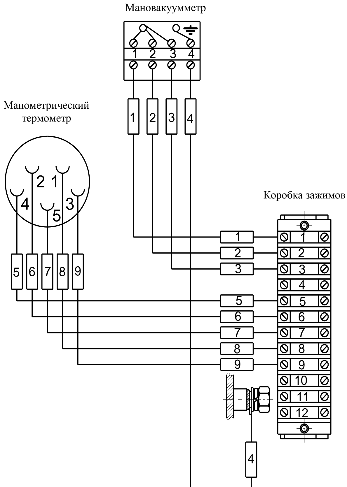
Рисунок 15 – Монтажная схема соединения коробки зажимов с контрольно-измерительными приборами
