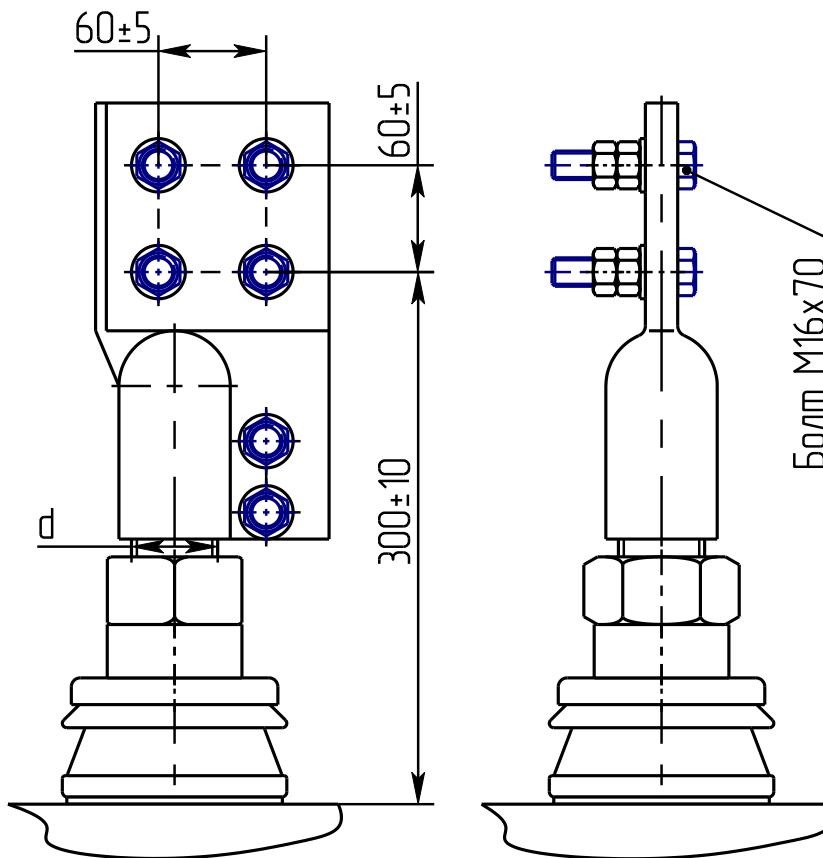
Рисунок 7 – Ввод НН на номинальный ток 2500 А
