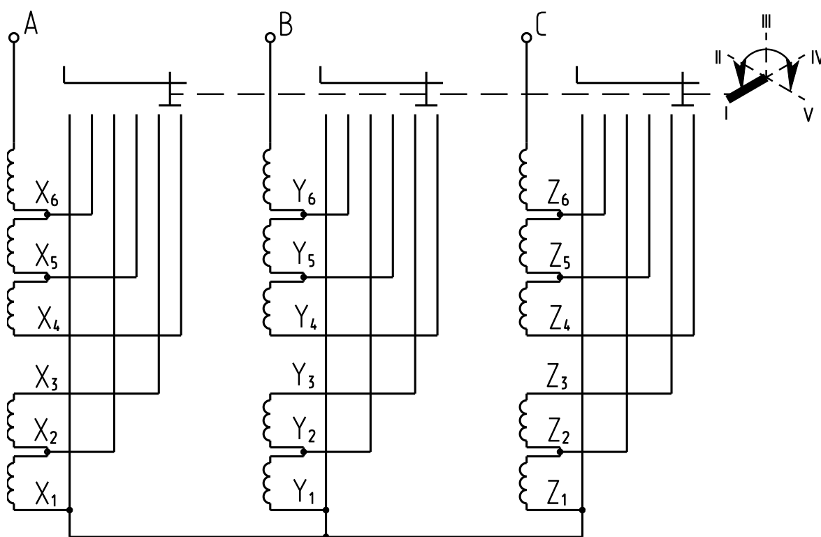
Рисунок 9 – Схема подсоединения ответвлений обмоток ВН к переключателю в трансформаторах мощностью 400 кВ·А при схеме соединения обмоток – «ЗВЕЗДА»
