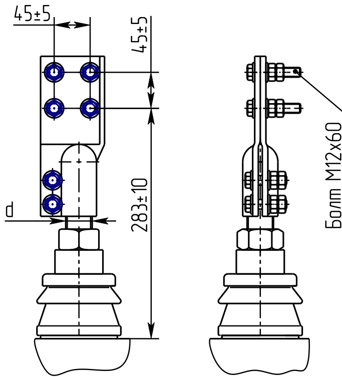
Рисунок 6 – Ввод НН на номинальный ток 1600 А
