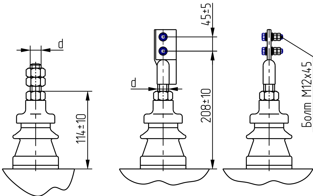
Рисунок 4 – Ввод НН на номинальные токи до 630 А
